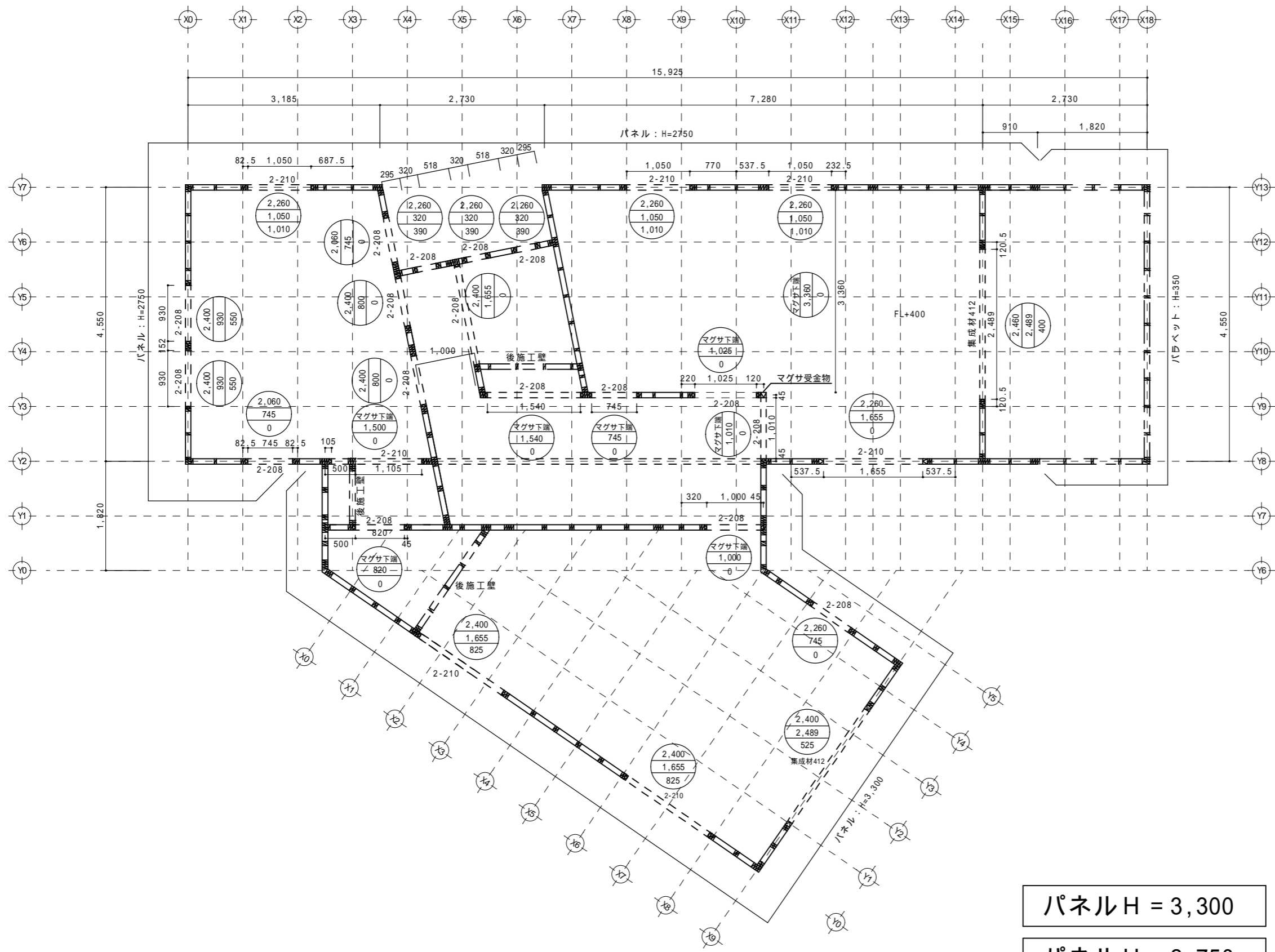
2階縦枠図 (1/50)
