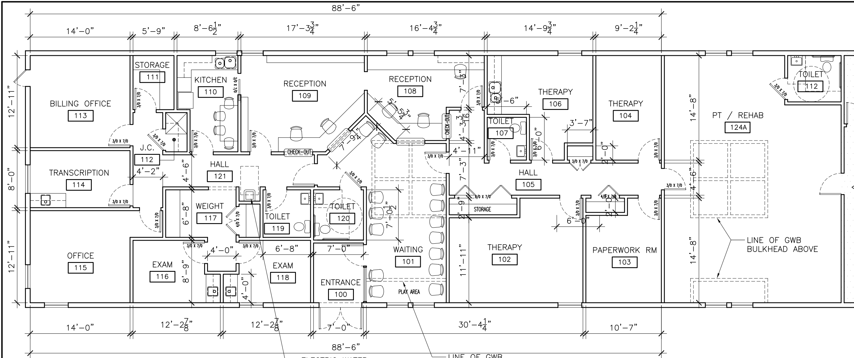
1 FLOOR PLAN SCALE: 1/8" = 1'-0"
